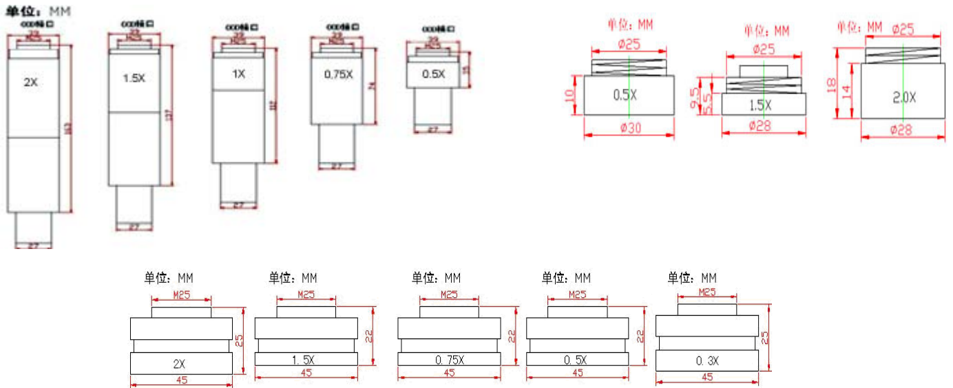
【ZL0910、ZL0911 工业镜头 CCD 接口和物镜外形尺寸】
